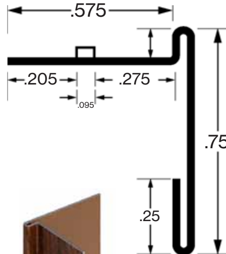
J Insert
